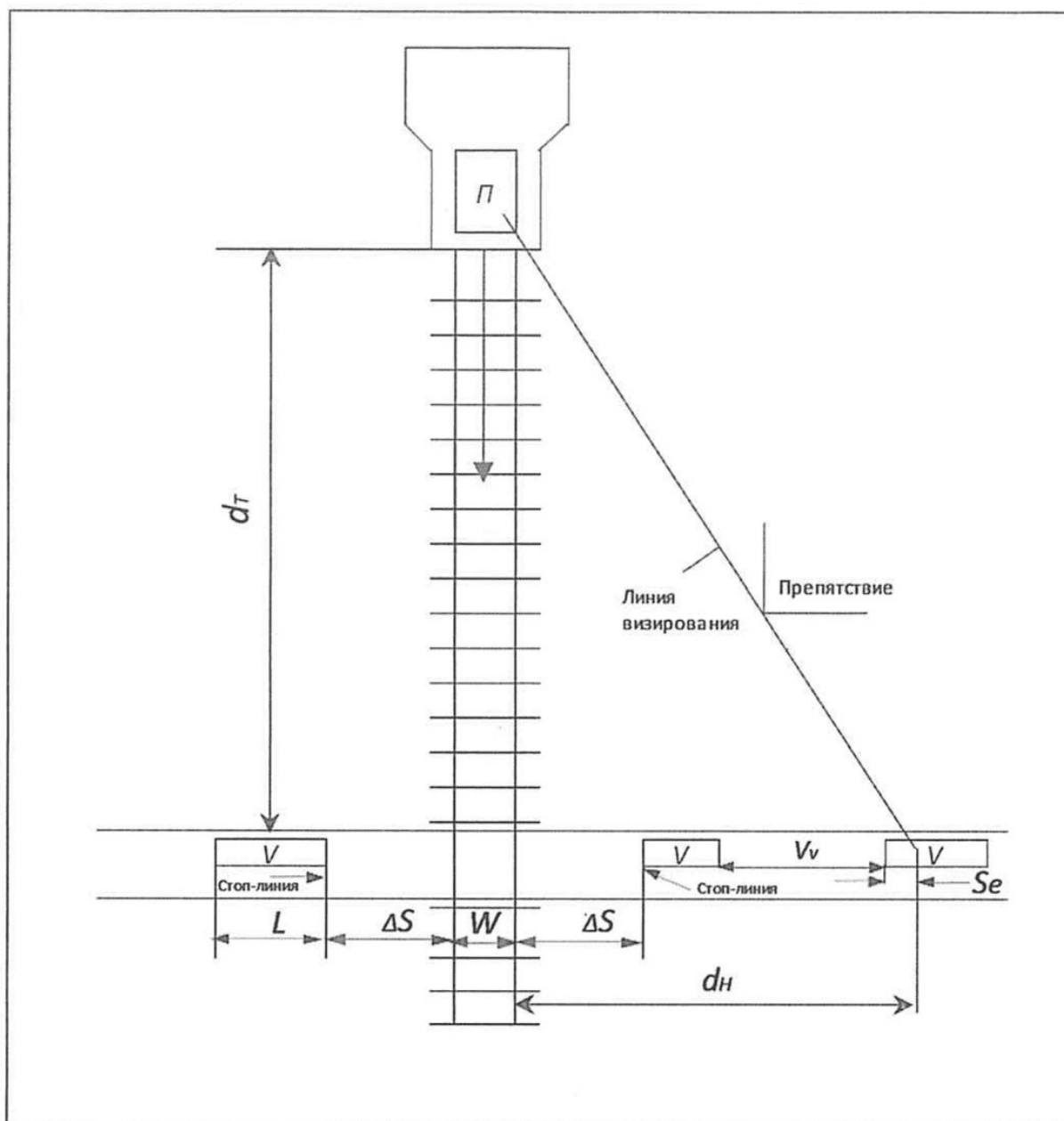
Рисунок К.1 - Схема определения расстояния видимости железнодорожного переезда (сигналов переездной сигнализации и шлагбаумов) вдоль автомобильной дороги d_n и расстояния видимости приближающегося к переезду поезда вдоль железнодорожных путей d_t
