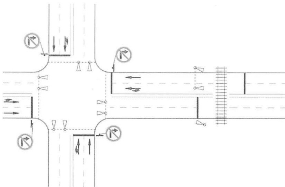
Рисунок К.4 - Схема размещения дополнительных светофоров
