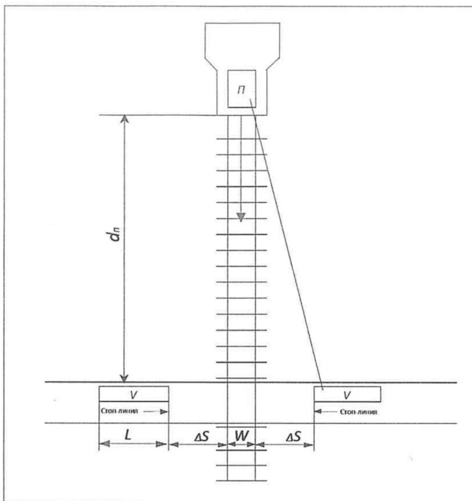
Рисунок К.2 - Схема определения расстояния видимости поезда из стоящего у железнодорожного переезда автомобиля
